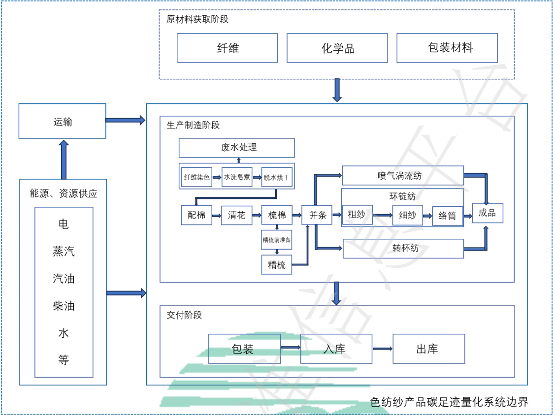
图 1 色纺纱产品碳足迹量化的系统边界示意图
