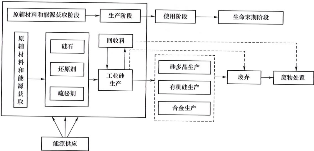
图 1 工业硅产品生命周期系统边界图
