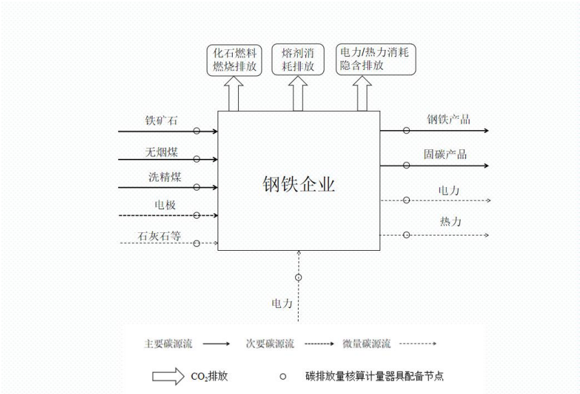
图 A.1 以法人为边界的钢铁企业碳源流图
