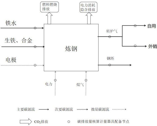
图 A.2 以工序为边界的碳源流图（炼钢）
